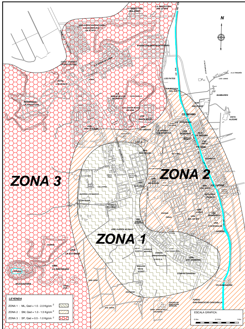
Fig. Nº 1: Zonificación Geotécnica
